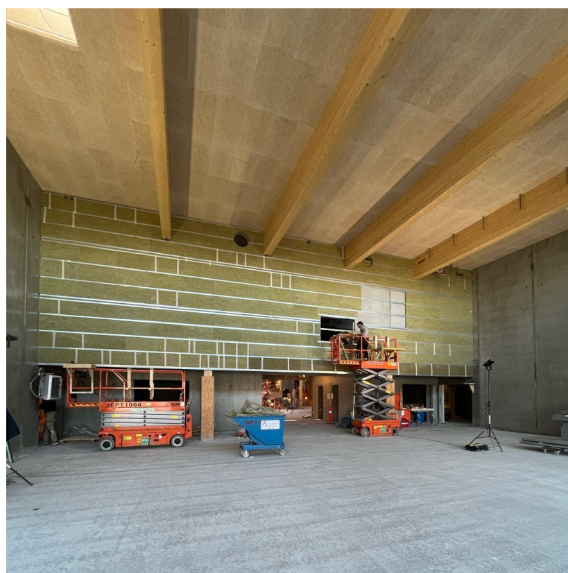
Figur 2: Foto af loftmontage og underlag for akustikbeklædning i multisal
